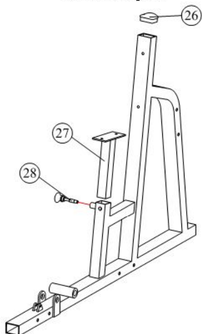
В. Главная рама
